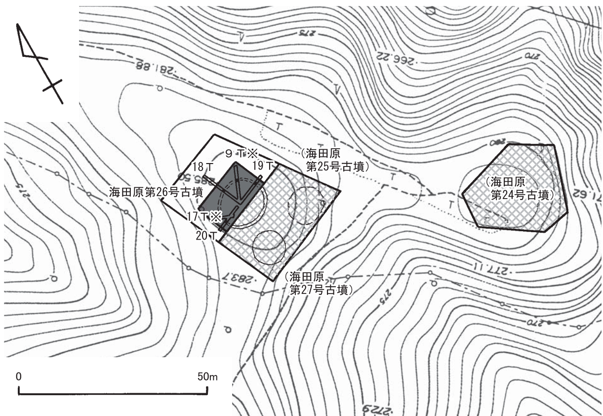
第7図 中国横断自動車道尾道松江線 海田原第25・27号古墳隣接地追加試掘範囲図（1：1,000） ※ 9 T・17 Tは平成20年度試掘坑の再発掘
