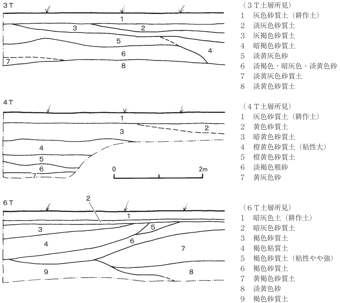
第14図 主要地方道呉環状線要試掘地点No.1 3 T東端南壁・4 T西端北壁・6 T西端北壁土層図 (1:50)
