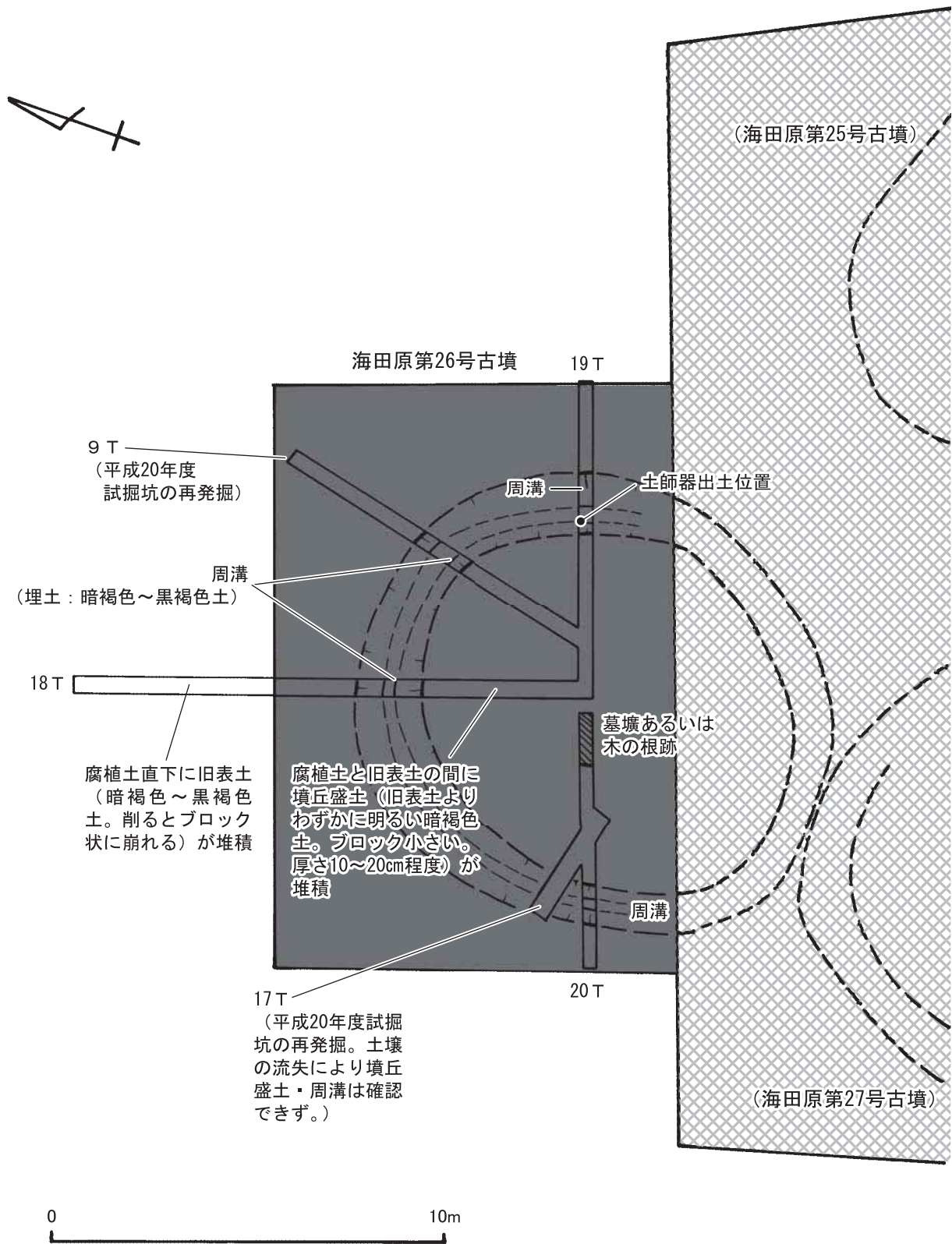
第8図 中国横断自動車道尾道松江線 海田原第25・27号古墳隣接地 試掘坑位置及び遺構略測図 (1:150)
